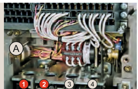
Fig. A: Piastra superiore del meccanismo Fig. B: Montaggio interblocco di rete: Fig. C: Montaggio interblocco di rete: Fig. D: Collegamento spinotti interblocco di rete: Fig. F: Posizioni interne
