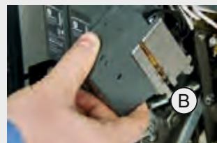
Fig. A: Piastra superiore del meccanismo Fig. B: Inserimento della bobina di sgancio a lancio di corrente Fig. C: Assemblaggio della bobina di sgancio a lancio di corrente Fig. D: Cablaggio Fig. E: Bobina con spinotto
