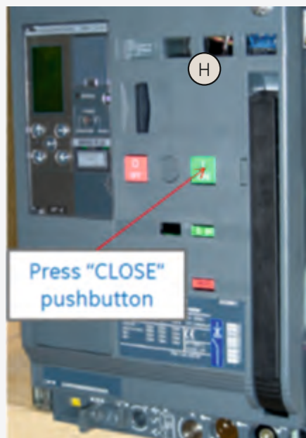
Abb. F: Zeigt den Versuch, die Handkurbelblende zu öffnen. Abb. G: Blockierter Sicherheitsriegel. Abb. H: Den "CLOSE"-Einschaltbaster betätigen um den Schalter einzuschalten (ON|EIN). Abb. I: "OFF"-Ausschaltbaster betätigen und den Schlüssel entnehmen.
