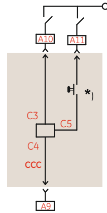
Connection scheme Command Closing Coil BLOCK A Anschlussschema Befehls-Abbrufmagnet BLOCK A Schema di connessione della bobina di chiusura a comando Morsettiara A
