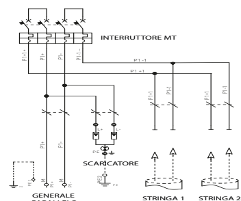
SCHEMA DI DUE STRINGHE DA DUPLICARE
