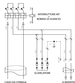
SCHEMA DI UNA STRINGA DA QUADRUPLICARE
