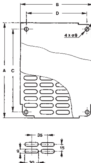
Piastra di fondo
