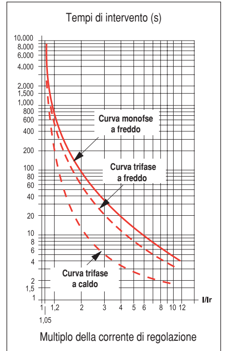
b90K Classe 10
