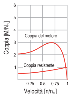
Curva Coppia-Velocità
