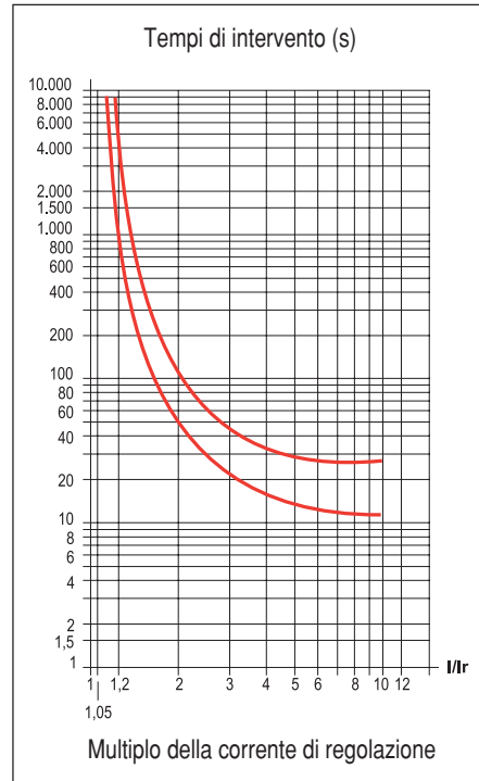
bw375K Classe 30
