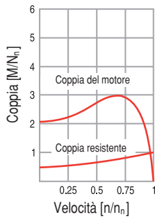
Curva Coppia-Velocità
