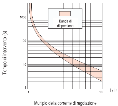
Curva di intervento (valori medi) con partenza da freddo
