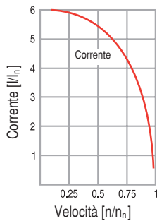
Curva Corrente-Velocità
