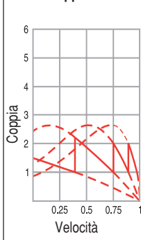
Curve Coppia-Velocità
