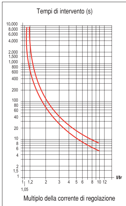
b450K Classe 10
