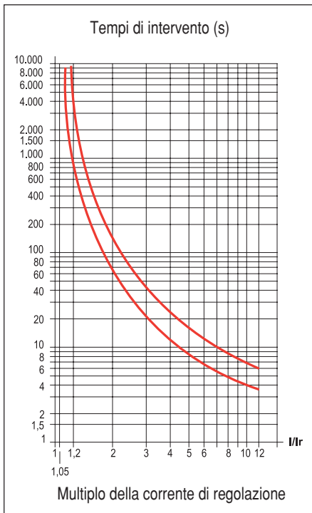
b160K Classe 10
