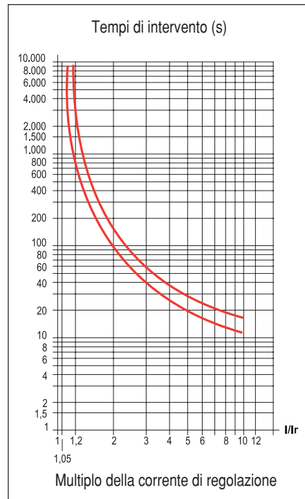
bw450K Classe 30
