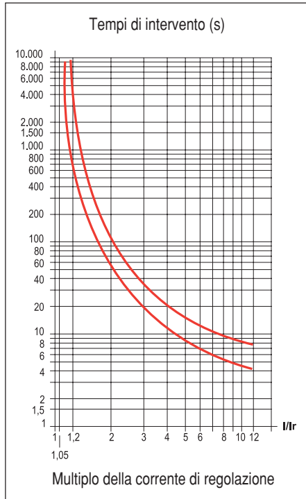
b375K Classe 10
