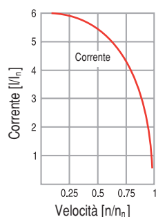
Curva Corrente-Velocità
