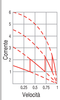
Curve Corrente-Velocità
